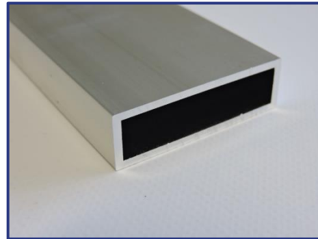
SX 50 versterking 50x15x2mm
