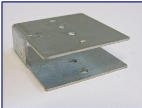
FIX 50 bevestiging versterking SX 50 op profiel
